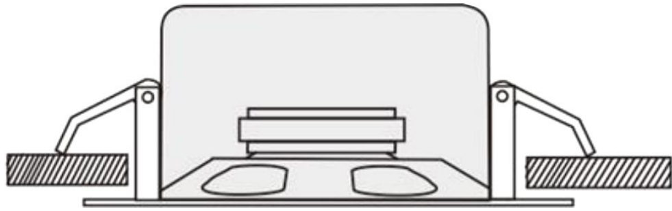
Рисунок 4 – Монтаж громкоговорителя
